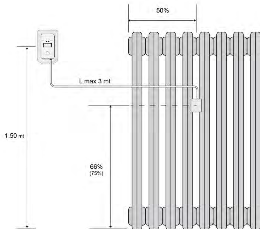
Figura 1. Punto di montaggio del ripartitore sul termosifone (sinistra), punto di montaggio del sensore remoto sul termosifone e del ripartitore a muro (destra).
