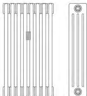
Tubular - Tubolare H >1200 mm
